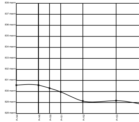
Escala Vertical 1:10 Escala Horizontal 1:100
