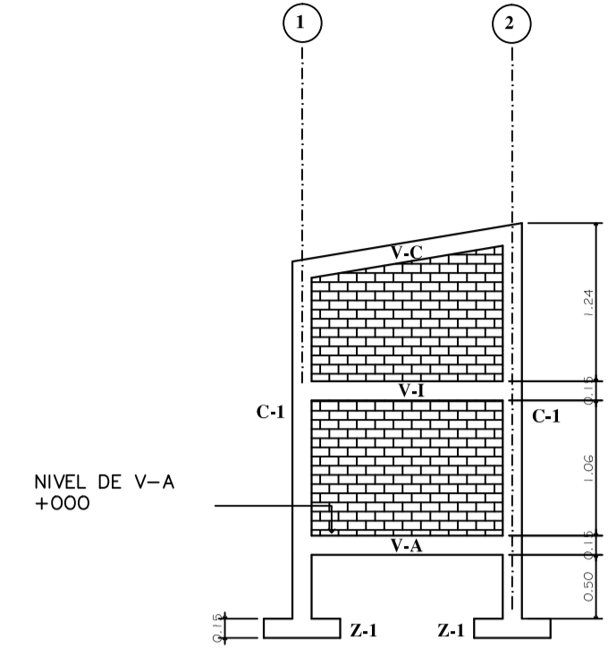
ELEVACION ESTRUCTURAL EJE B
