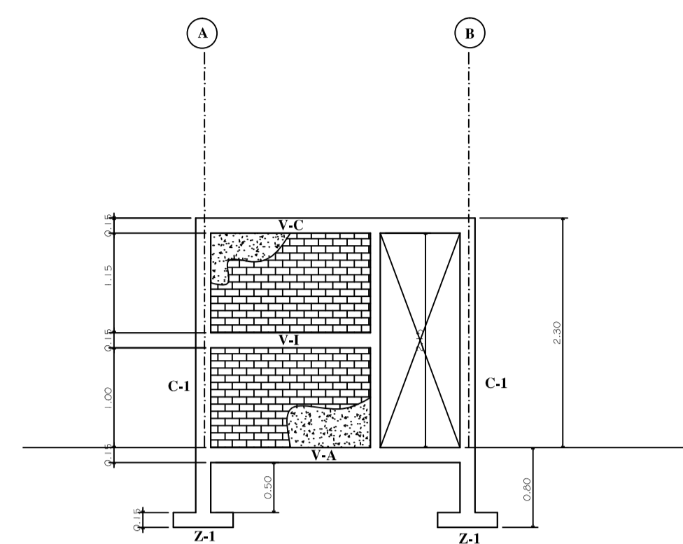
ELEVACION ESTRUCTURAL EJE 1
