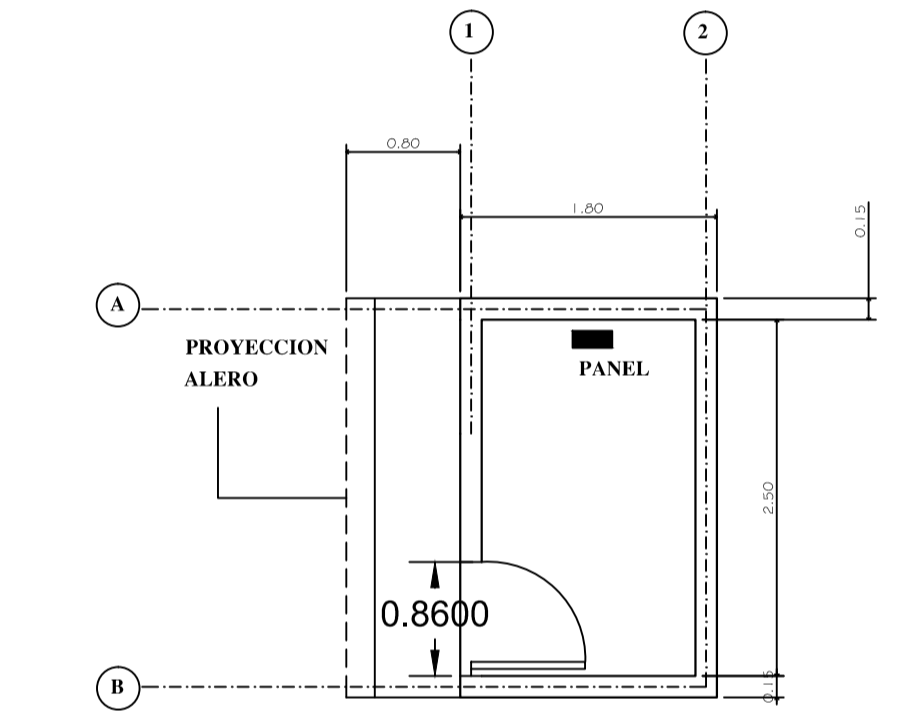
PLANTA ARQUITECTONICA CASETA DE CONTROL
