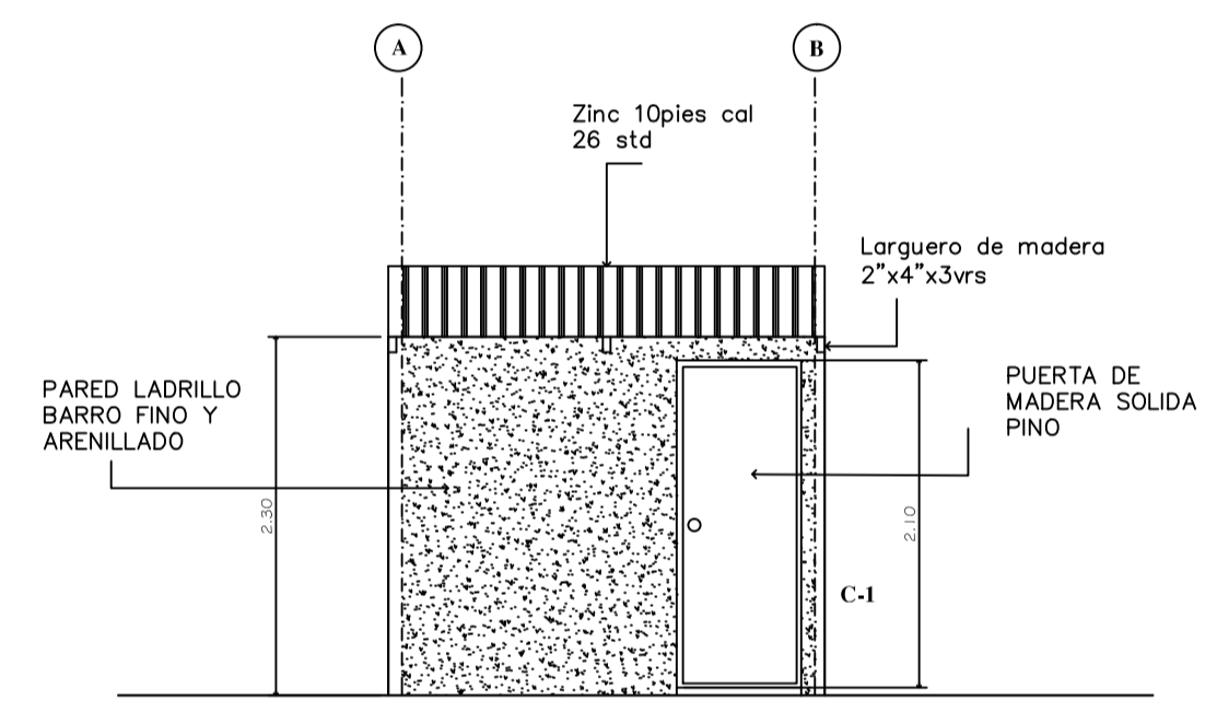
ELEVACION CASETA DE CONTROL EJE 1
