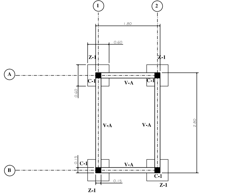
PLANTA DE FUNDACION
