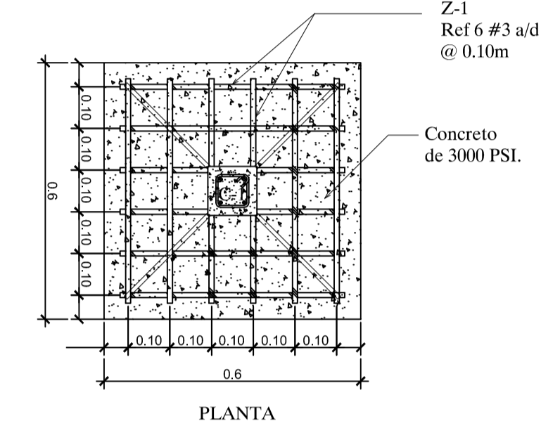
DETALLE DE ZAPATA Z-1
