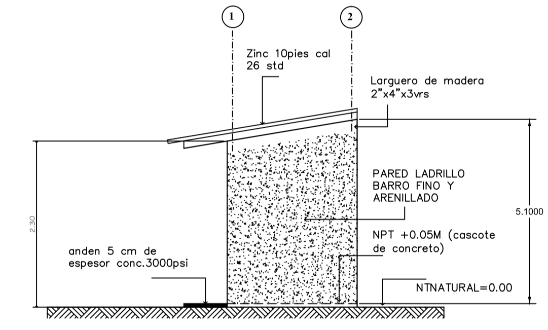
ELEVACION CASETA DE CONTROL EJE B
